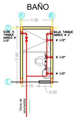
PLANTA INSTALACION HIDRÁULICA
