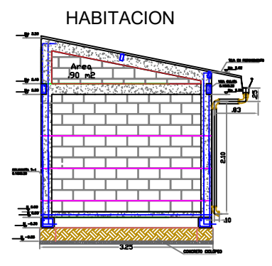
DETALLE BAJANTE AGUAS LUVIAS
