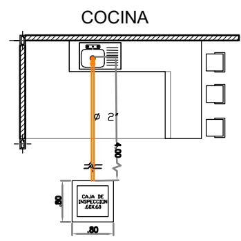
PLANTA INSTALACION SANITARIA
