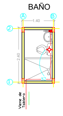
PLANTA INSTALACION ELÉCTRICA
